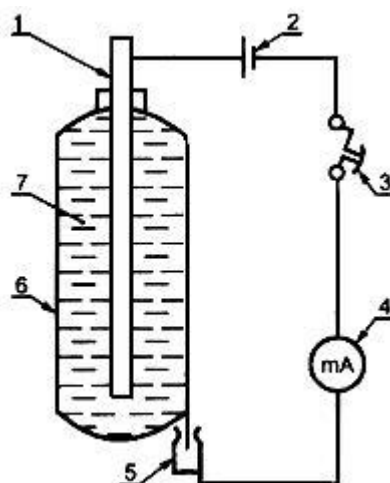
Рисунок 2 - Схема проверки целостности внутреннего покрытия корпуса огнетушителя
